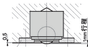
倒置安装说明
